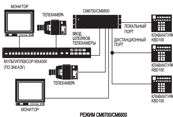
РЕЖИМ CM6700/CM6800
