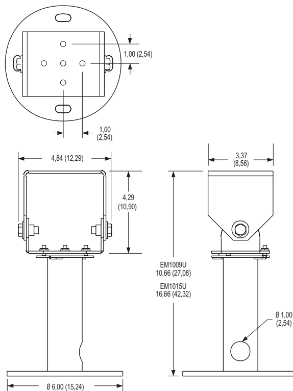
РАЗМЕРНЫЙ ЧЕРТЕЖ EM1009U/EM1015U
