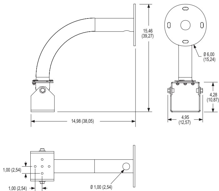
РАЗМЕРНЫЙ ЧЕРТЕЖ EM1900U
